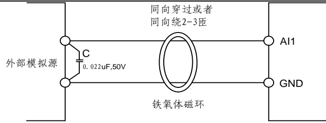
图 3-12 模拟量输入端子处理接线图
