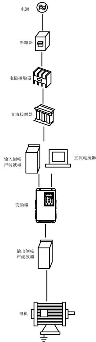
图 3-2 AE300 变频器与外围机器的连接示例
