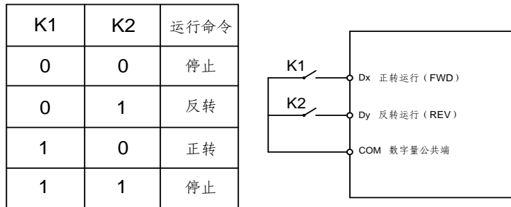
图 6-5 两线式模式 1
