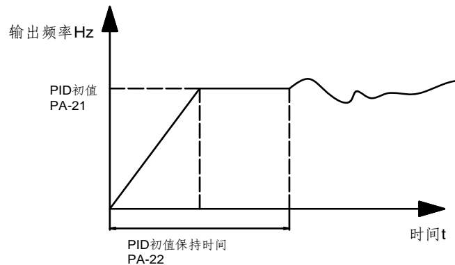
图 6-26 PID 初值功能示意图
