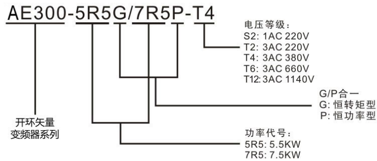
图 2-1 型号说明
