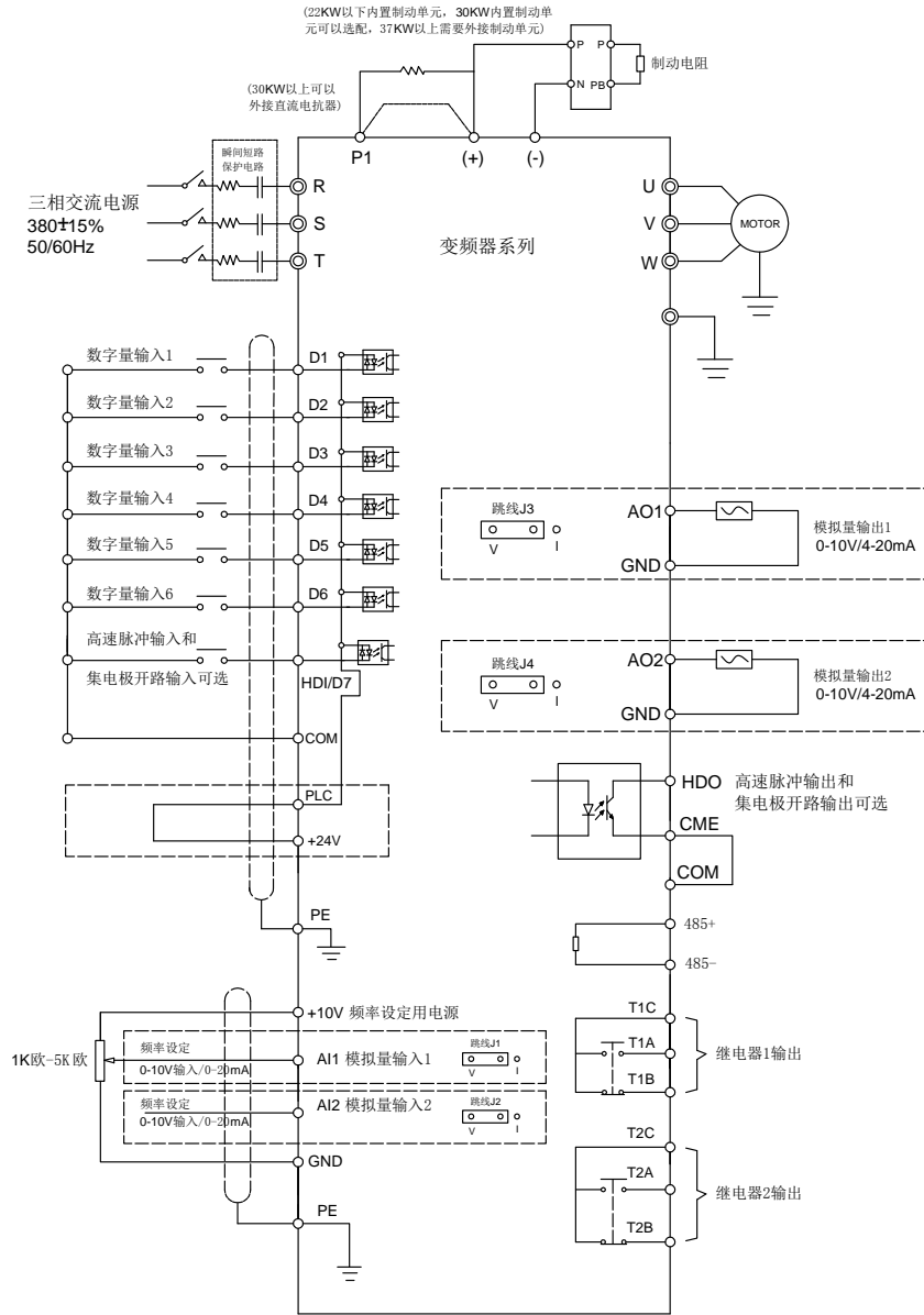
图 3-3 接线图
