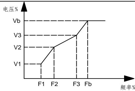
V1-V3: 多段速V/F第1-3段电压百分比 F1-F3: 多段速V/F第1-3段频率百分比 Vb:电机额定电压 Fb:电机额定运行频率
