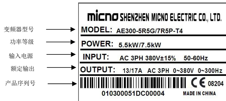
图 2-2 铭牌说明
