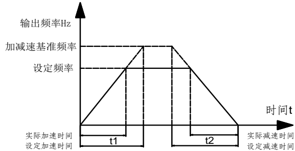
图 6-1 加减速时间示意图
