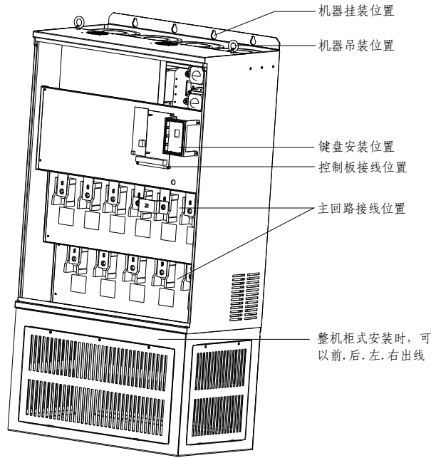
图 2-3 变频器各部件说明
